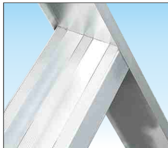
Gradini profondi 83 mm. molto robusti saldati su spessori maggiorati Unito al montante verticale mediante robusta saldatura ad angolo nascosta alla vista, a garanzia della massima stabilità e di lunga affidabilità nel tempo
