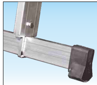
Basetta stabilizzatrice ad innesto calibrato indeformabile con montaggio e smontaggio rapido Di facile montaggio, scarica le sollecitazioni sul profilo garantendo la massima solidità nel tempo
