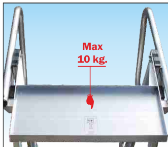
Grande vaschetta porta-oggetti ribaltabile con portata fino a 10 kg. Ripiano di dimensioni mm. 200 x 550 ribaltabile per il trasporto realizzato in alluminio anti-ruggine, permette un sicuro appoggio per gli attrezzi
