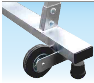
Basetta posteriore AUTO-FRENANTE con ruote per il trasporto a carriola Realizzata in alluminio è smontabile per il trasporto ed utilizza ruote in gomma nera Ø 125 mm. e tamponi a terra che frenano la scala automaticamente
