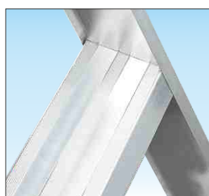
Gradino antiscivolo profondo 83 mm. accoppiato al montante con robusta saldatura ad angolo nascosta vista
