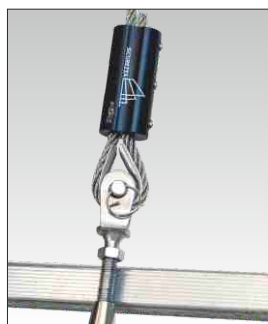
Occhiello di blocco fune a fissaggio regolabile
