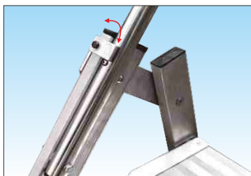
Parapetto realizzato con tubo Ø 32 mm. in alluminio ribaltabile ad aggancio rapido
